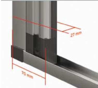
Ingombro manigliette
