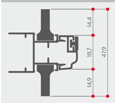
Ingombro manigliette
