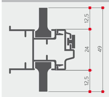
Ingombro con manigliette
